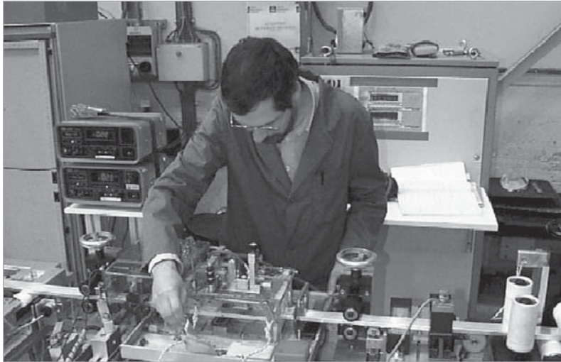
Ultraschall Phased Array Prüfung an einem koextrudierten Hochstrom-Supraleiterkabel
