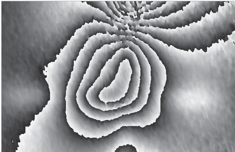
Gefiltertes Phasendifferenzbild ( 2\pi ) einer einseitig eingespannten Platte mit auf der Rückseite kreuzweise aufgetragenen Nuten unter punktueller Temperaturbelastung
