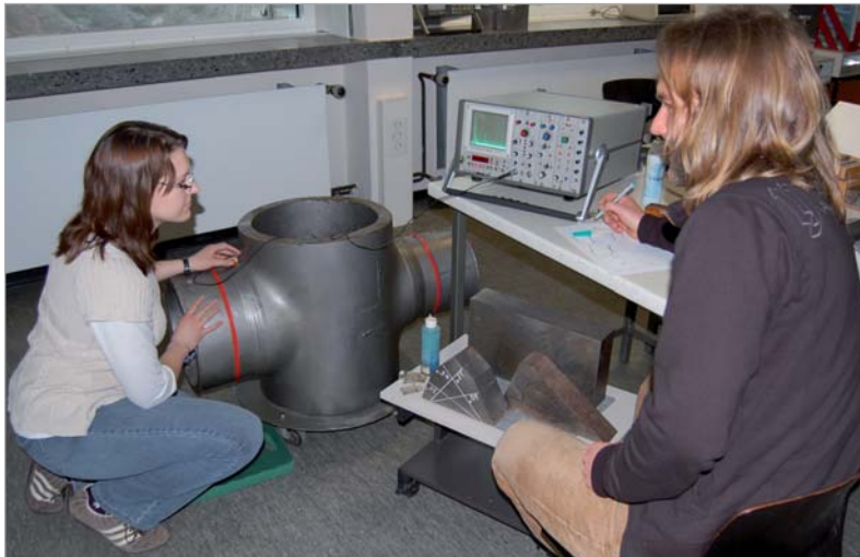
US-Praktikum, Untersuchung auf Rissbildung durch Thermoschock
