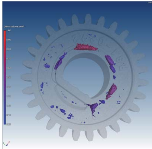
Defektanalyse an einem Zahnrad
