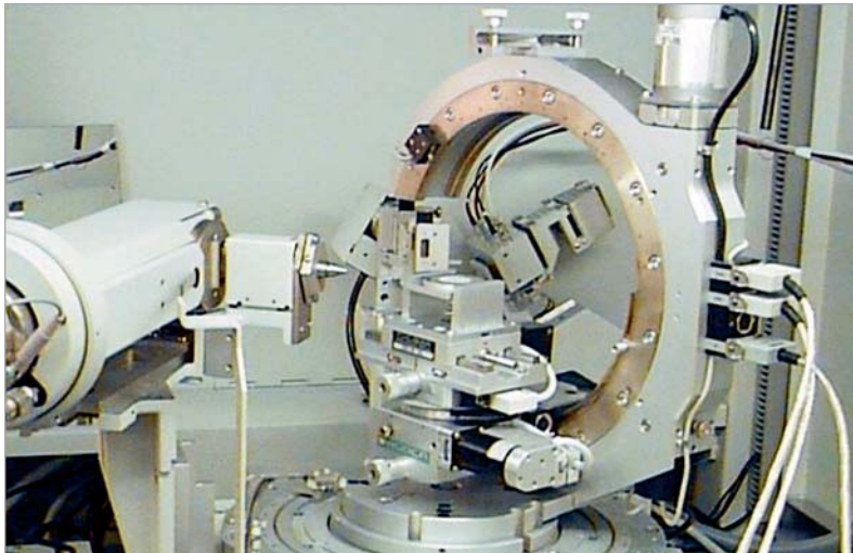
Röntgendiffraktometer mit Eulerwiege zur röntgenographischen Spannungs- und Texturmessungsmessung
