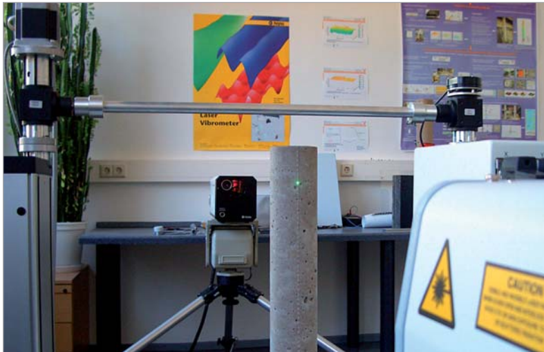
Linienscan mit Laser-Ultraschall zur Beurteilung der Sedimentationsstabilität an einem Zylinder aus Selbstverdichtendem Beton (SVB)
