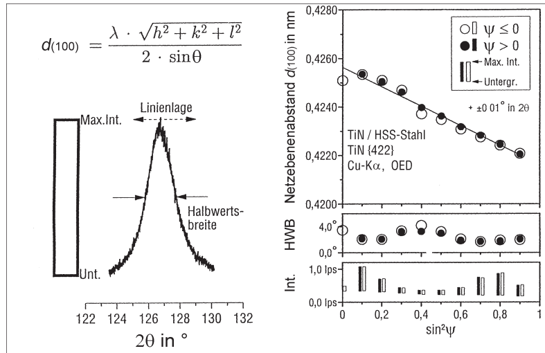
Beispiel für die Auswertung von Röntgeninterferenzlinien zur Ermittlung der Eigenspannung in einer Werkstoffoberfläche.
