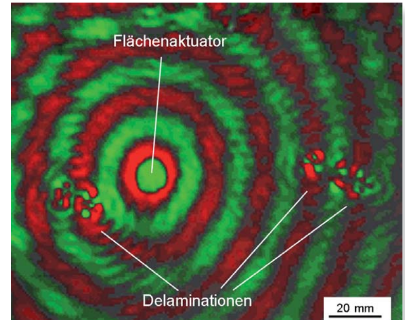
Ausbreitung von Lambwellen in einer CFK-Platte und Wechselwirkung mit Delaminationen (Quelle: M. Krüger, Diplomarbeit, Otto-von-Guericke-Universität Magdeburg)
