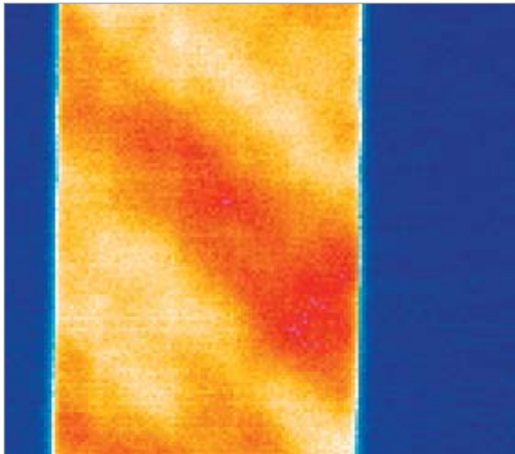
Oberflächentemperaturverteilung auf einem dynamisch belasteten textilverstärkten Kunststoff
