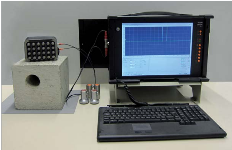
Computergesteuerte Ultraschallprüfeinrichtung
