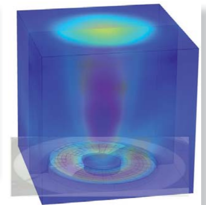
Schallfeldsimulation von Luftschallprüfköpfen
